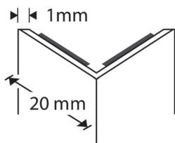
20 x 20 mm Kulmasuojalista | Hörnskyddsprofil | Corner protection
