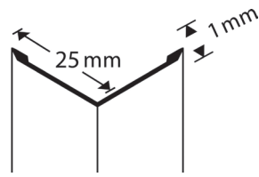
25 x 25 mm Kulmasuojalista | Hörnskyddsprofil | Corner protection
