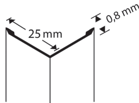
25 x 25 mm Kulmasuojalista | Hörnskyddsprofil | Corner protection
