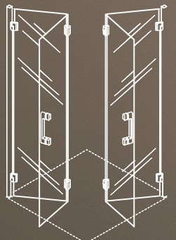
90x90x195 cm Ante a libro Accordion doors
