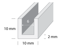
U-lista
