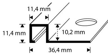
Laattalista H= 10 mm valkoinen
