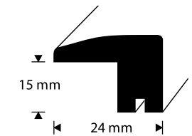
Päätelista, tammi 15 x 24 mm, 100 cm ja 200 cm
