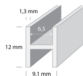
H-lista
