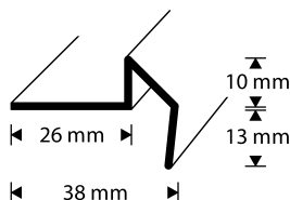
Laatta-askelkulmalista RST
