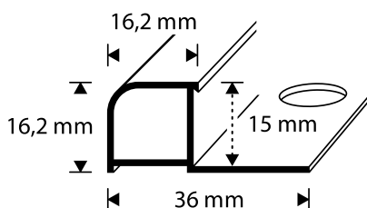
H=15 mm Pyöreä | Rund | Circular
