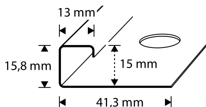
H=15 mm Avoin neliö | Öppen kvadrat | Open square
